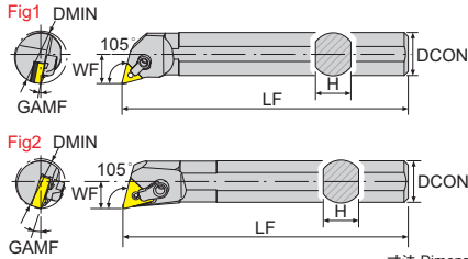
寸法 Dimension(mm)
