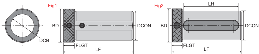
寸法 Dimension(mm)
