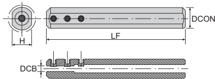
寸法 Dimension(mm)
