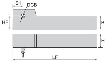
寸法 Dimension(mm)
