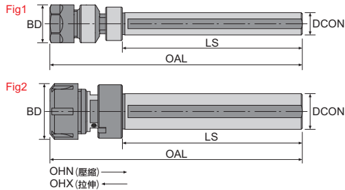
寸法 Dimension(mm)
