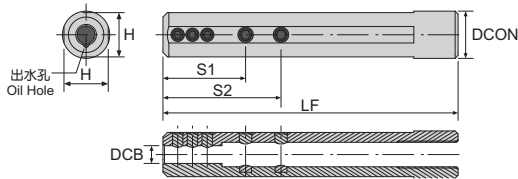
寸法 Dimension(mm)
