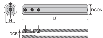
寸法 Dimension(mm)
